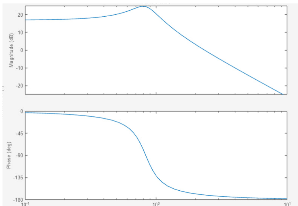
Рисунок 10 – ЛАЧХ и ЛФЧХ колебательного звена
